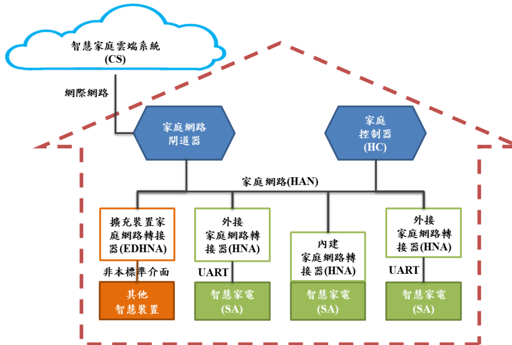
圖 1. TaiSEIA 101 智慧家庭網路通訊架構
